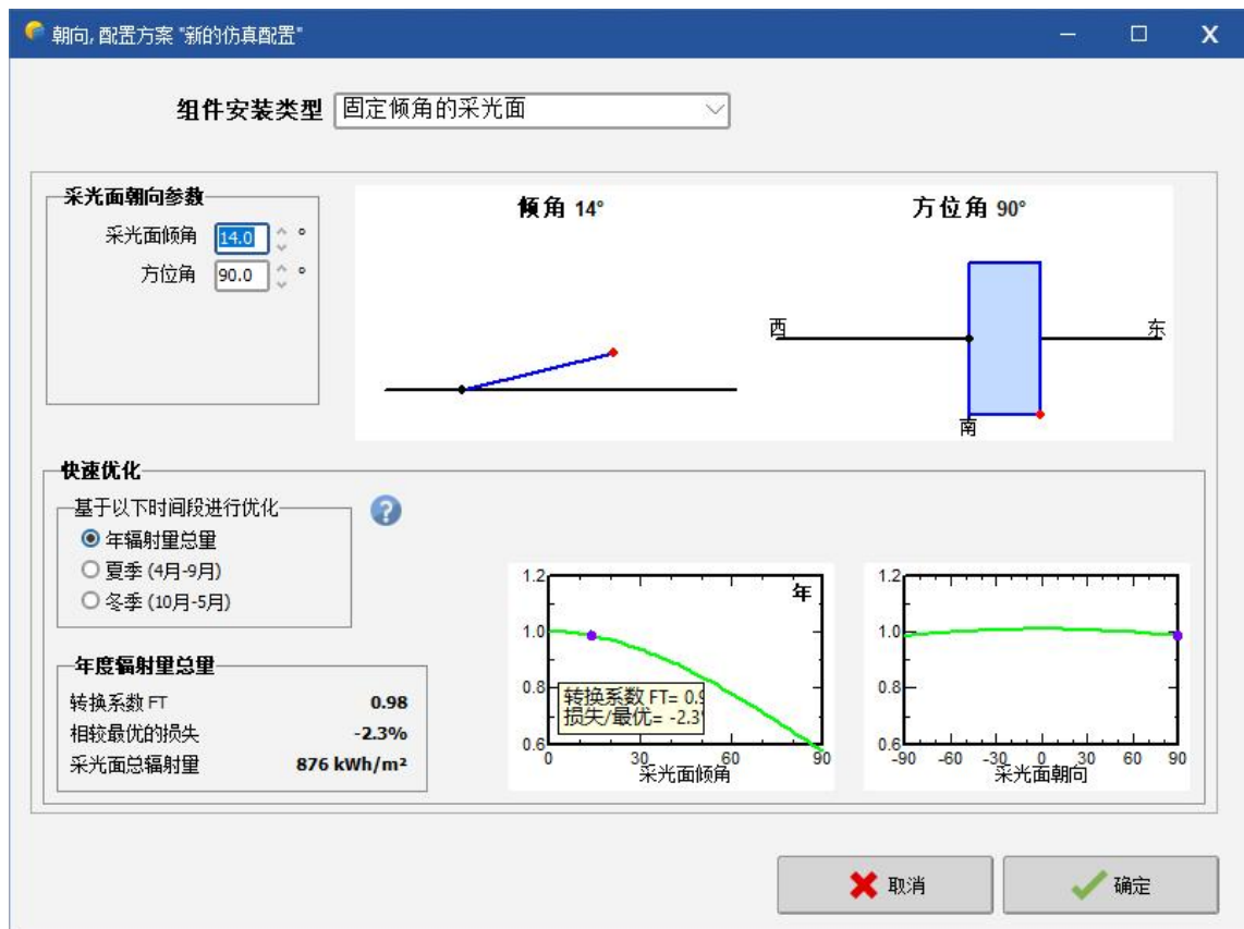
图5.5-4厂房顶光伏组件倾角辐射量计算结果
