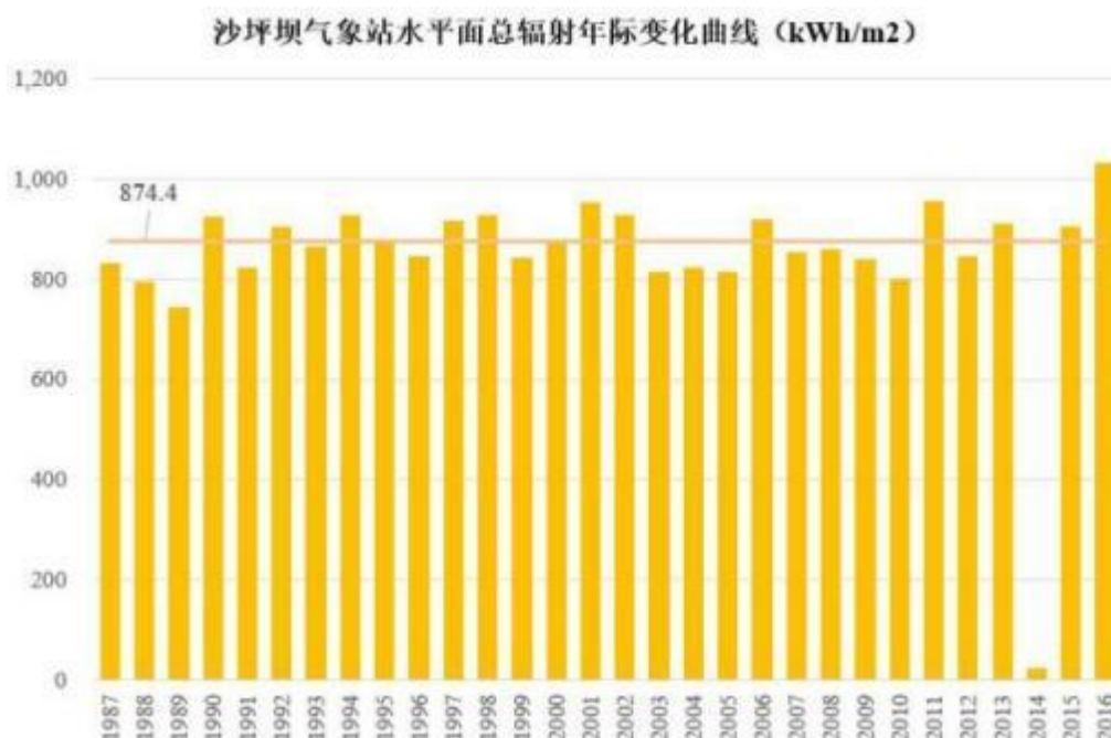
图2. 2-2沙坪坝气象站辐射量年际变化曲线(kWh/m 2 )
