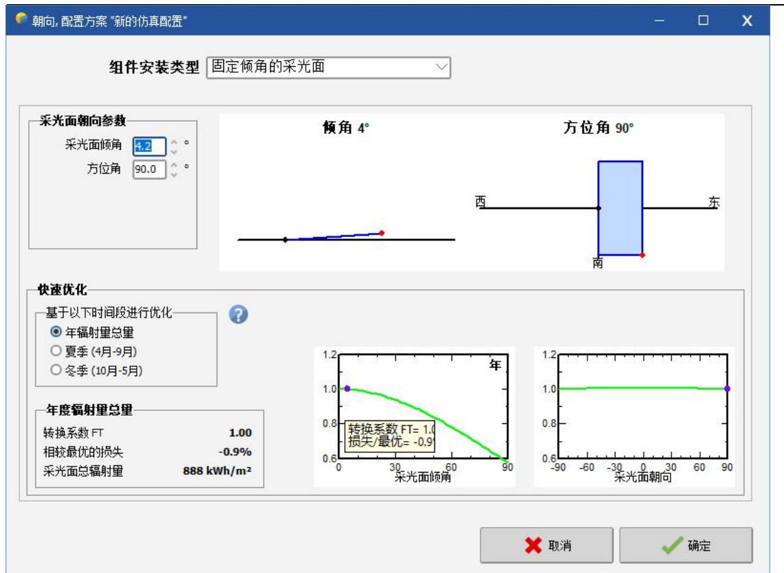
图5.5-3光伏车棚光伏组件倾角辐射量计算结果
