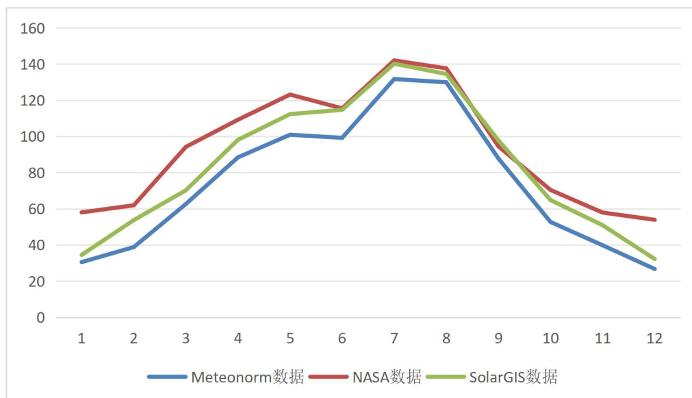
图2.2-4Meteonorm和NASA、SolarGIS逐月总辐射曲线（kWh/m²）
