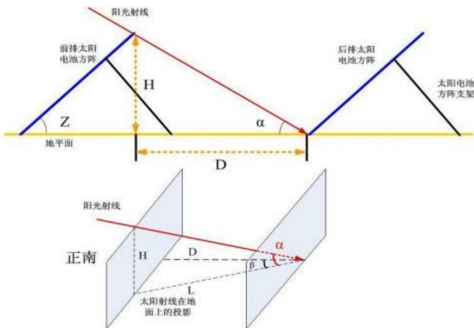
图4.5-4光伏阵列间距离示意图
